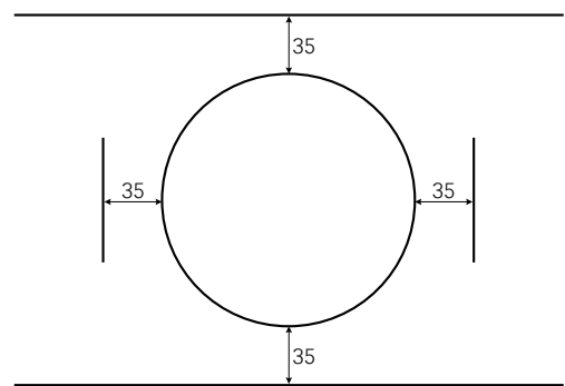
Mindestabstände für die Montage (Angaben in mm)
